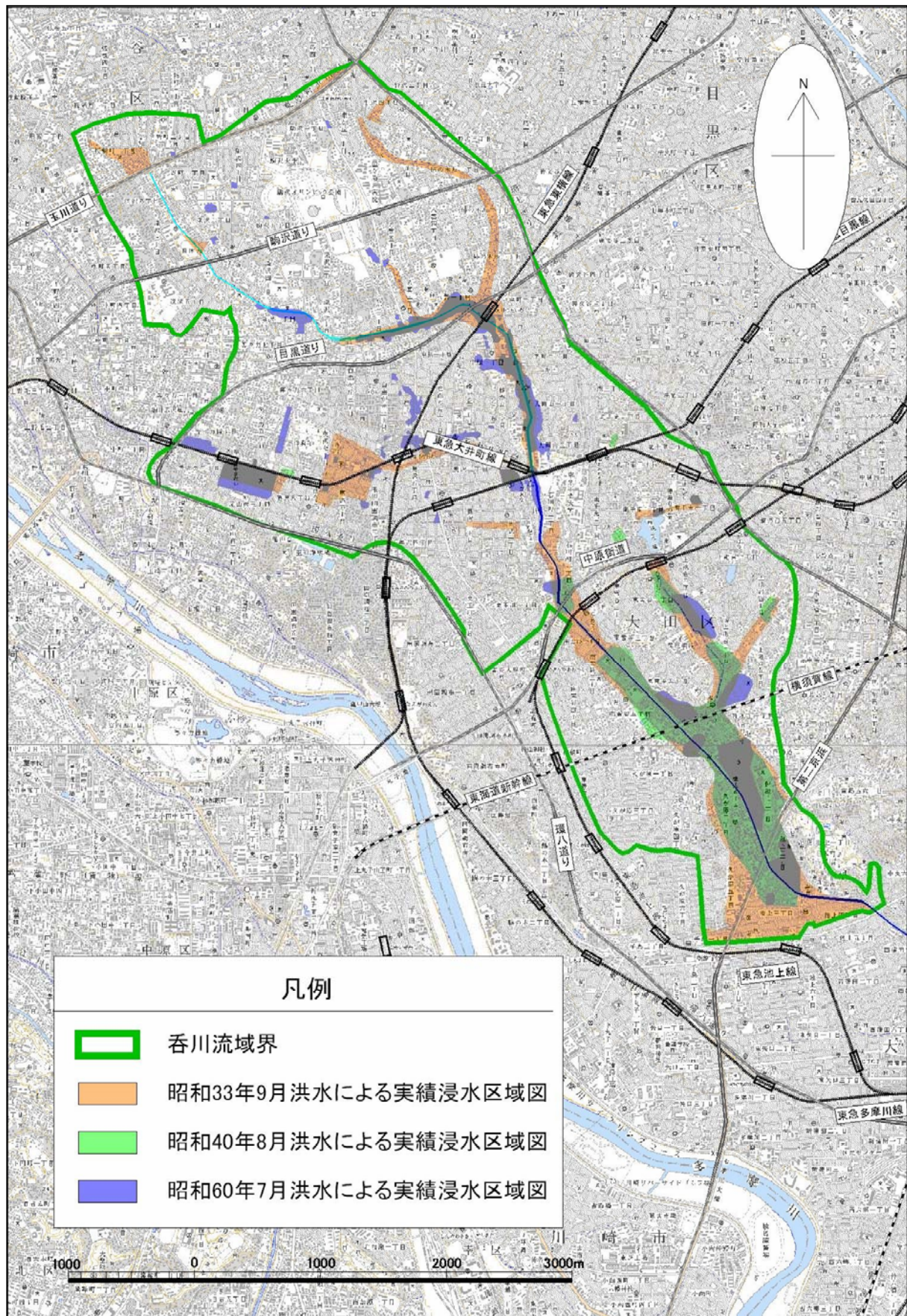
図 2-2 吞川流域浸水実績図
