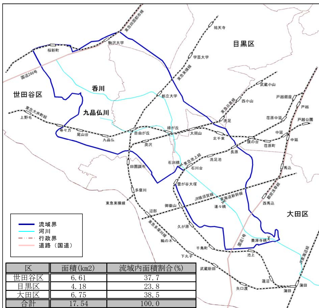
図 2-1 呑川流域概要図
